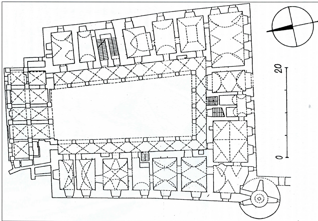
Půdorys přízemí zámku před rekonstrukcí.
