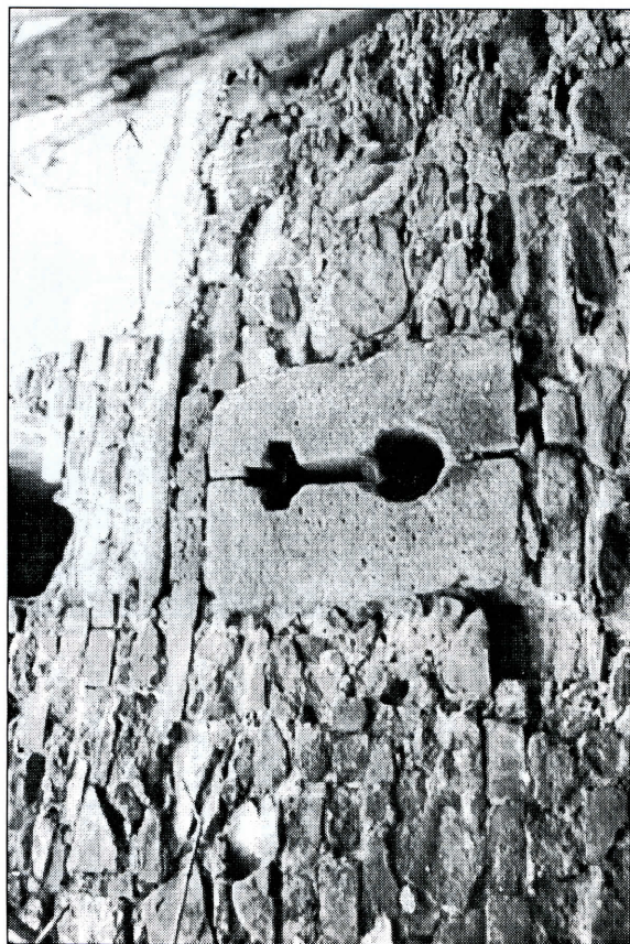
Křížová klíčová střílna v okrouhlé věži perštejnského hradu.
